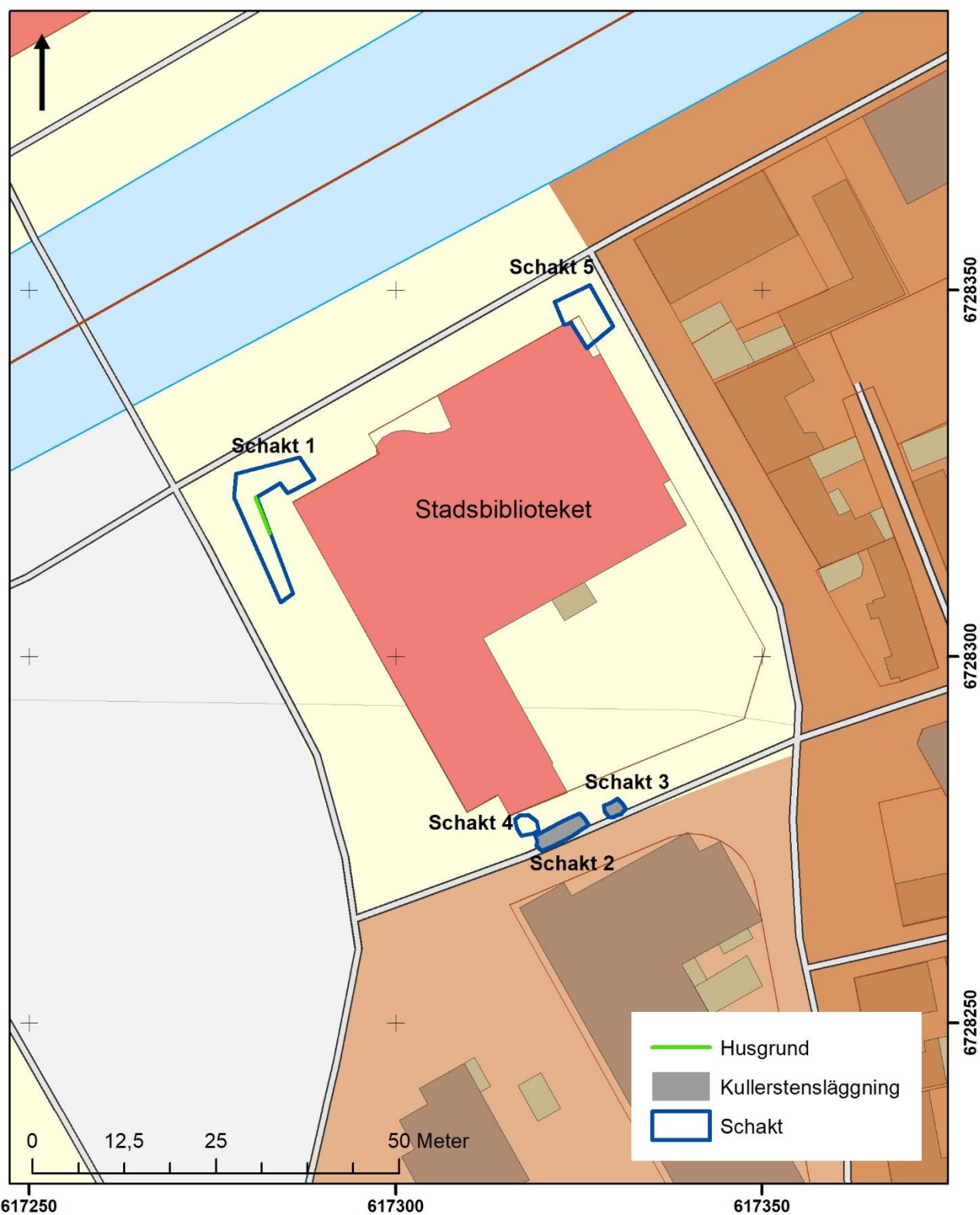
Figur 1. Schaktplan på utdrag ur Lantmäteriets fastighetsregister. Skala 1:800.
